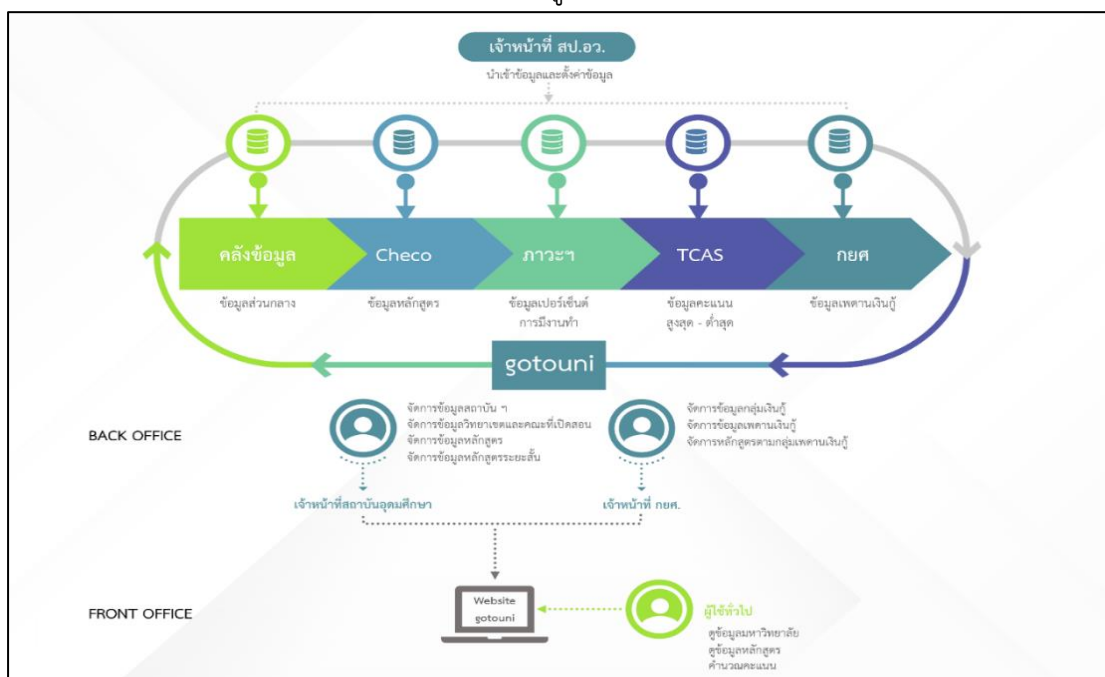
ภาพที่ ๑ - ๑ แผนภาพขั้นตอนการทำงานของระบบ
